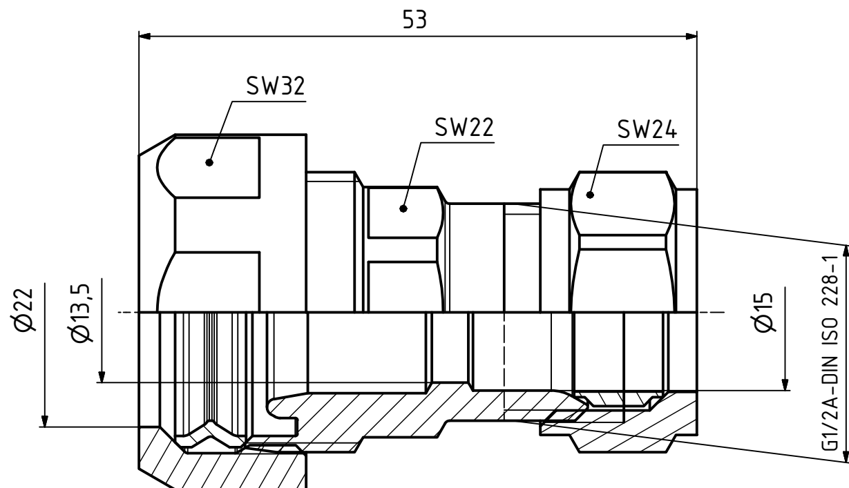
ÜG-Stück Cu Klemmverschraubung Ø15 x DN16 Art.-Nr.: 342860
