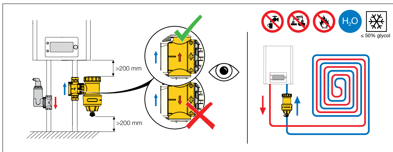
Abbildung 7: Positionierung
