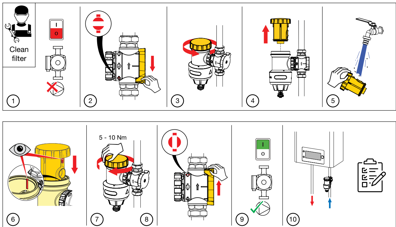
Abbildung 10: Filterreinigungsverfahren
