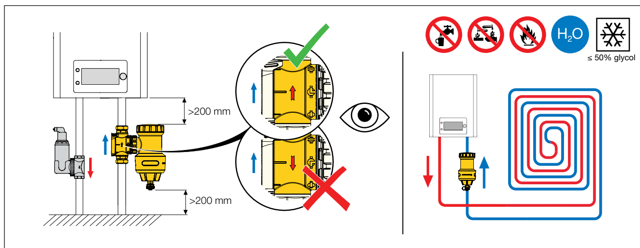
Figure 7: Positionnement
