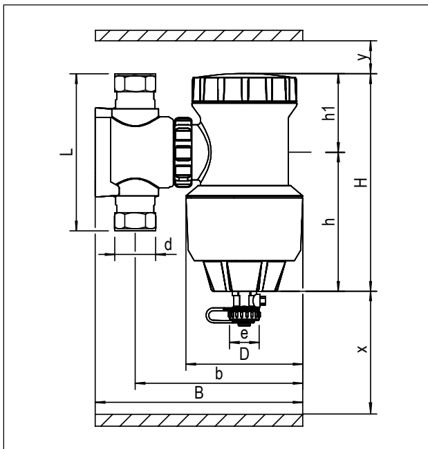
Abbildung 5: Maßzeichnung Abmessungen
