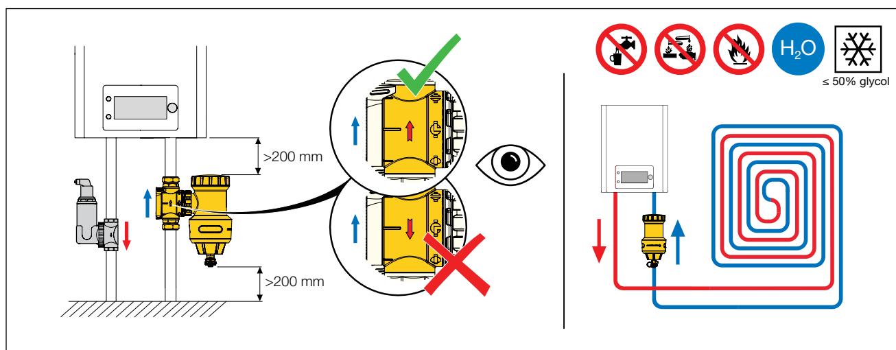
Figuur 7: Positionering
