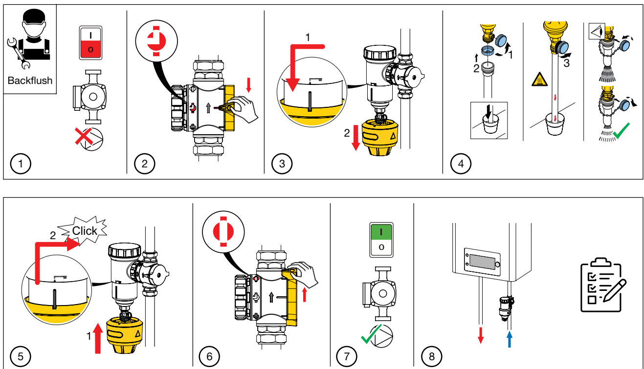
Abbildung 9: Rückspülverfahren
