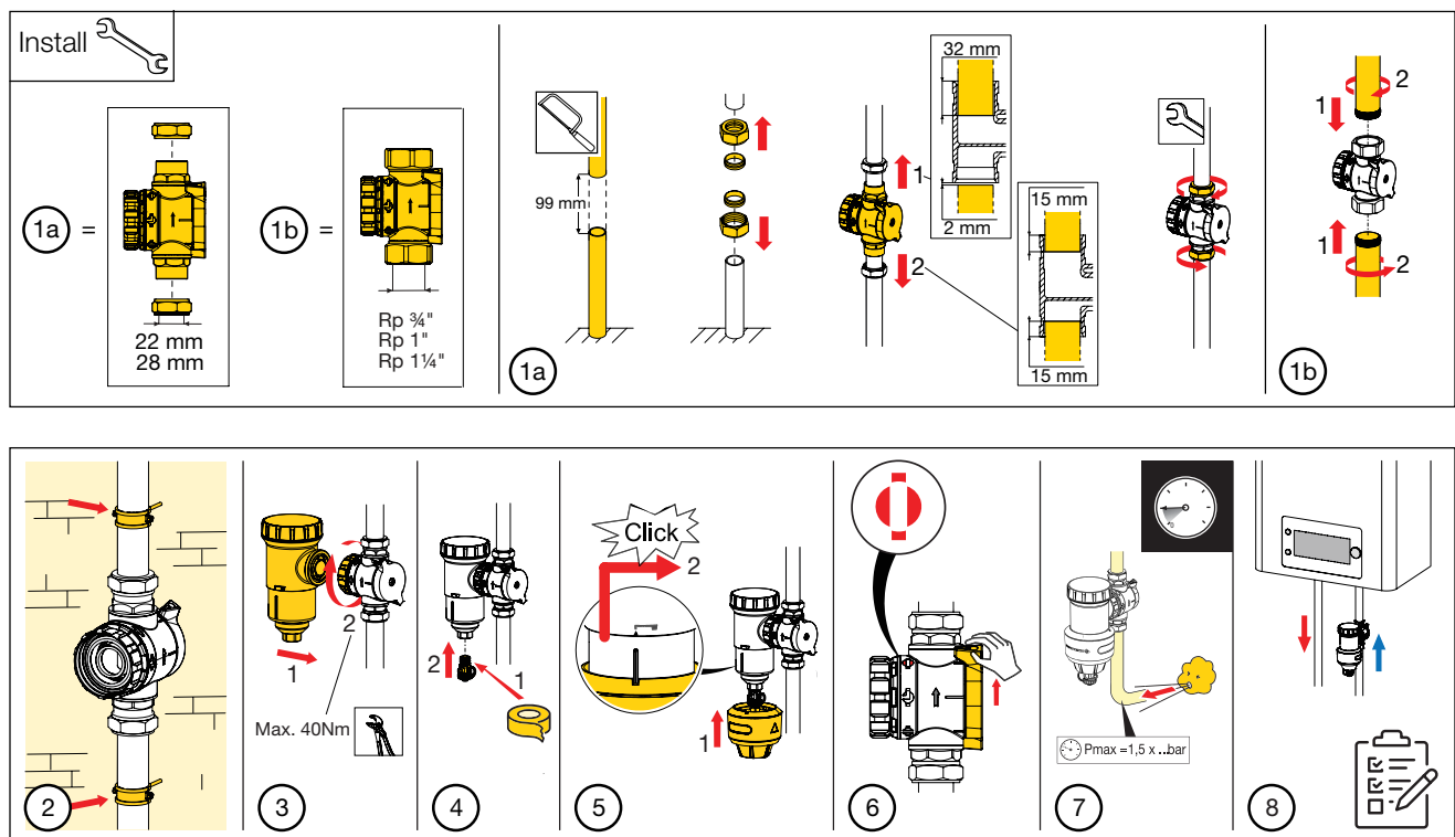
Figuur 8: Installatie
