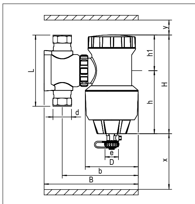
Figura 5: Dimensioni (disegno quotato)
