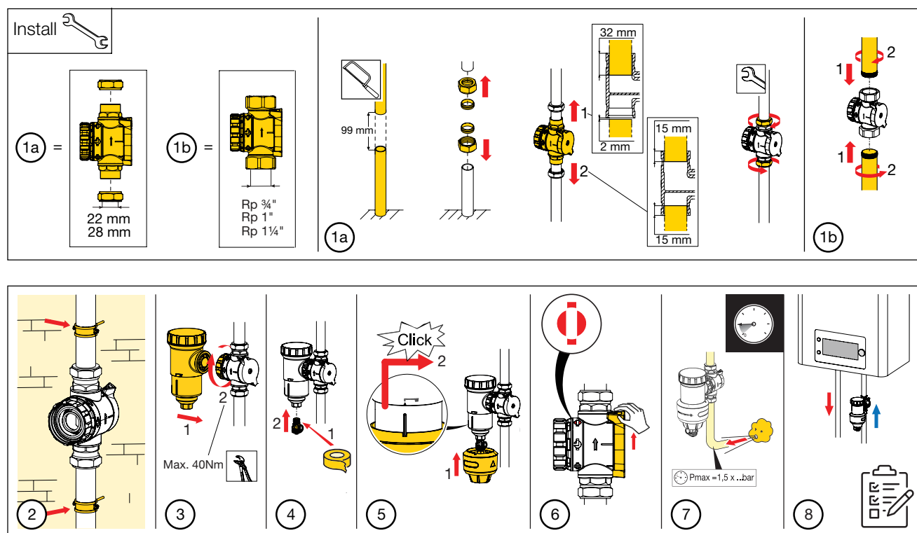
Figura 8: Installazione
