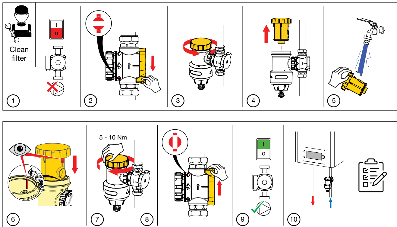
Figuur 10: Filterreinigingsprocedure
