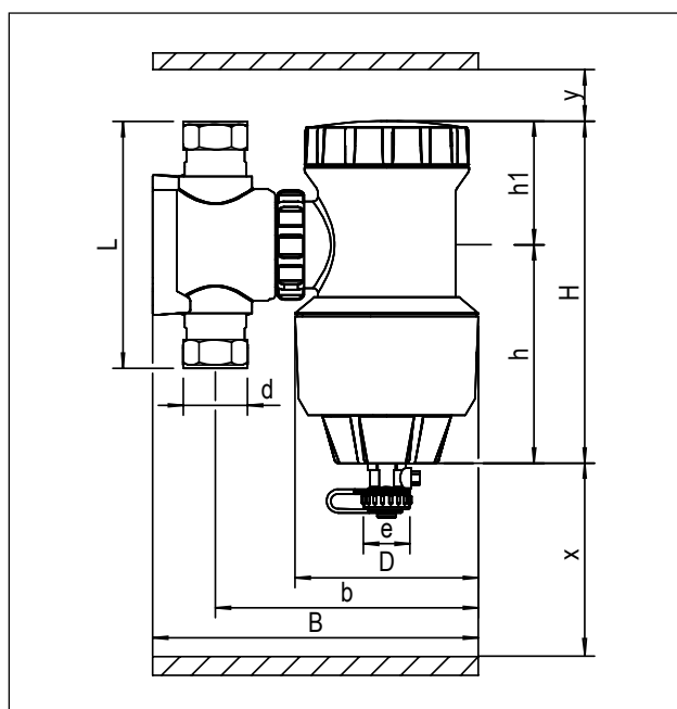
Figure 5: Dimensions du schéma coté
