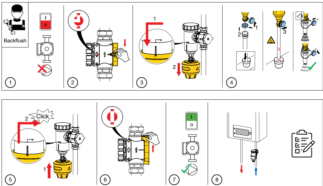
Figuur 9: Terugspoelprocedure
