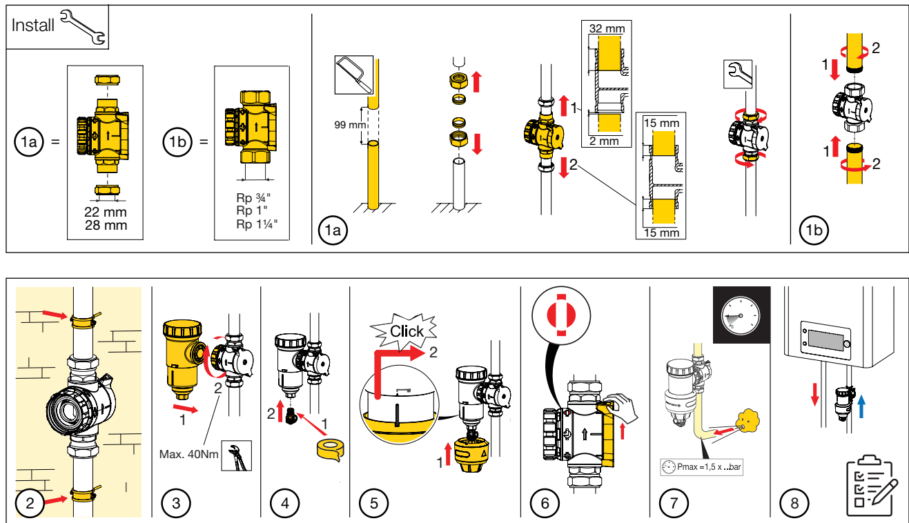
Abbildung 8: Installation
